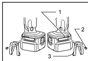
1. Ranura 2. Tornillo 3. Gancho
