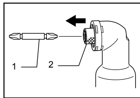
1. Punta 2. Base de mandril
