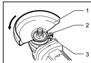
1. Protector (guarda) de disco 2. Caja de cojinetes 3. Tornillo
